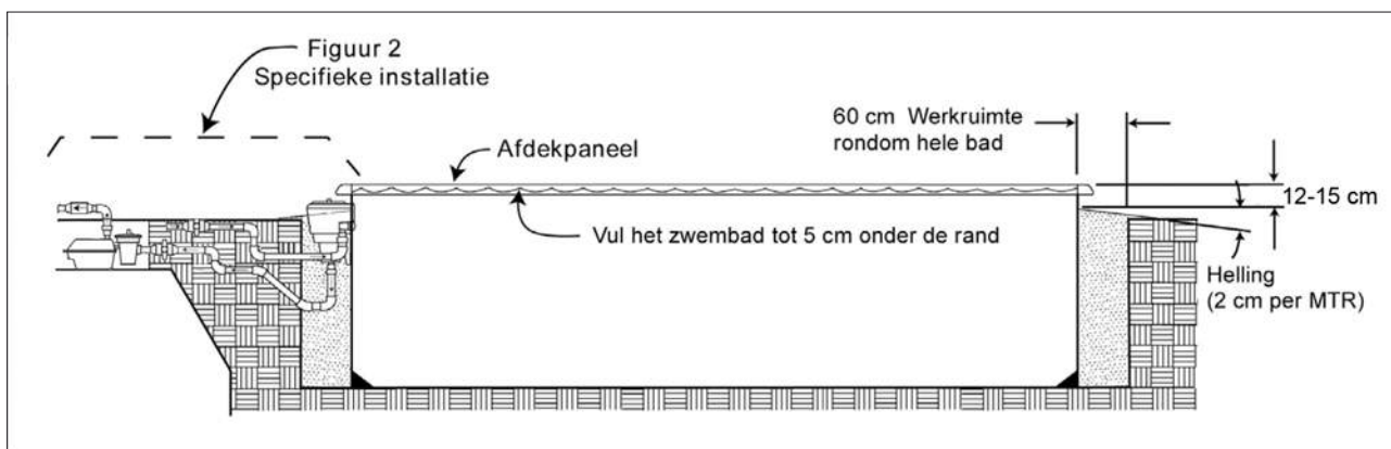
FIG. 1 - BOUWKUNDIGE VOORZIENINGEN WANNEER EEN ZWEMBAD WORDT INGRAVEN
